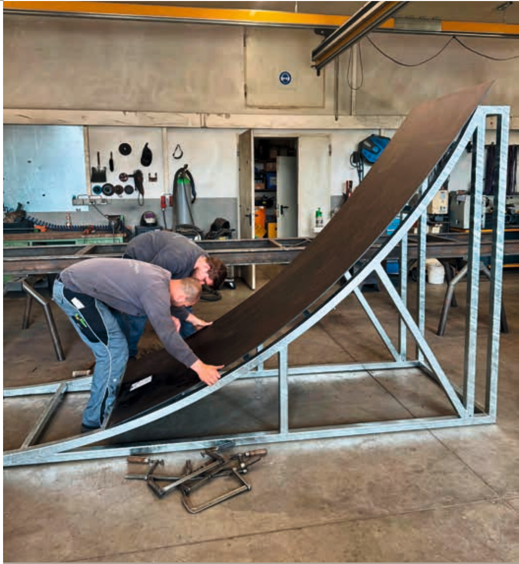
Skatesmart Belag wird auf Metallabsprung angebracht
